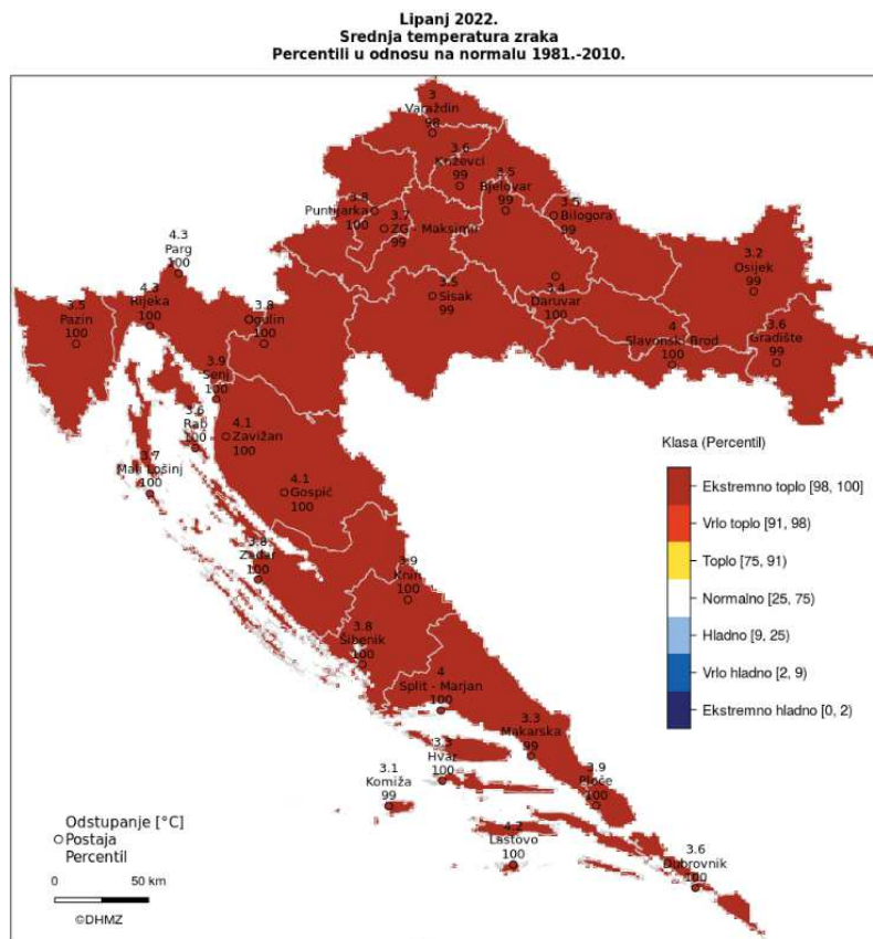
Slika 4. Odstupanje srednje mjesečne temperature zraka za lipanj 2022., DHMZ
