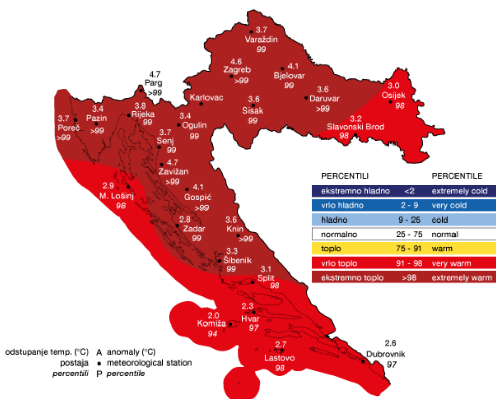
Slika 1. Odstupanje srednje mjesečne temperature, lipanj 2019., DHMZ
