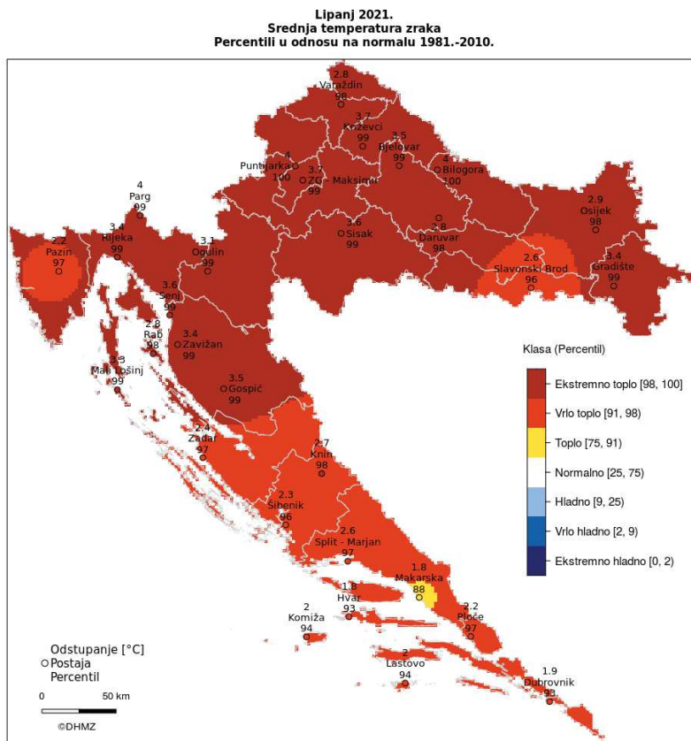
Slika 3. Odstupanje srednje mjesečne temperature, lipanj 2021., DHMZ
