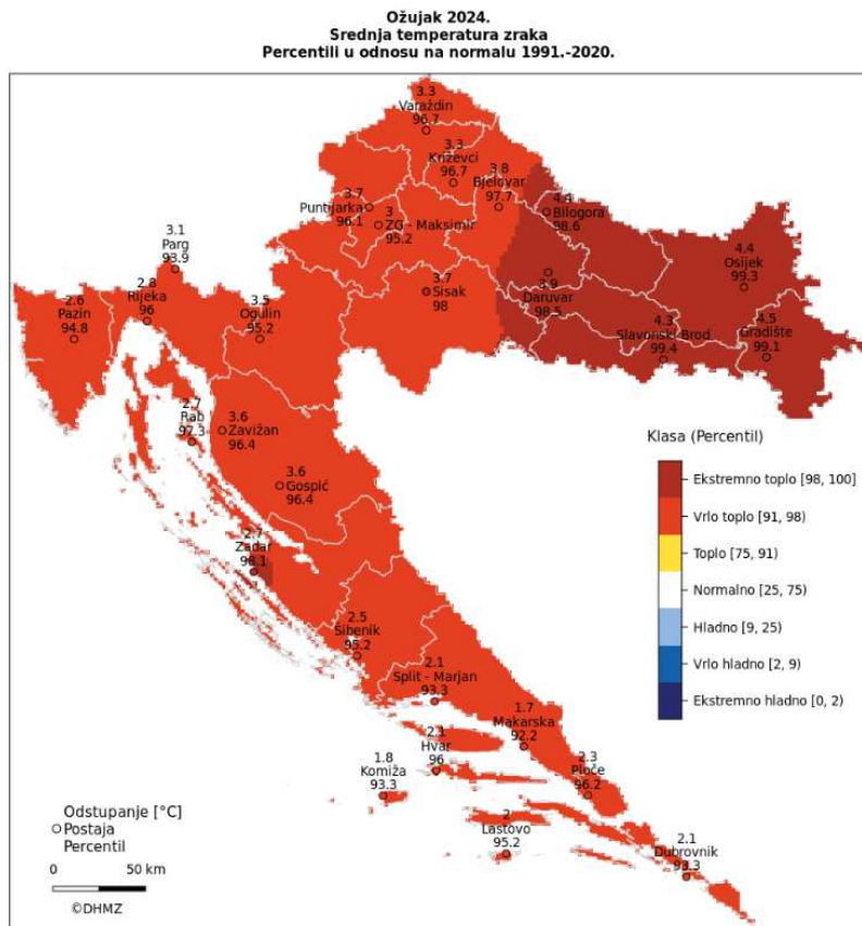
Slika 10. Odstupanje srednje mjesečne temperature zraka za ožujak 2024., DHMZ
