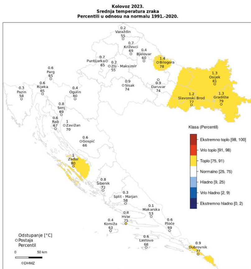
Slika 8. Odstupanje srednje mjesečne temperature zraka za kolovoz 2023., DHMZ
