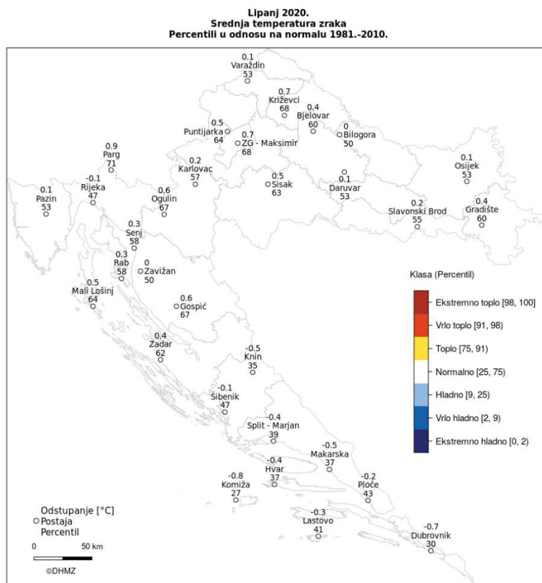
Slika 2. Odstupanje srednje mjesečne temperature, lipanj 2020., DHMZ
