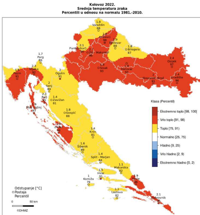
Slika 6. Odstupanje srednje mjesečne temperature zraka za kolovoz 2022., DHMZ
