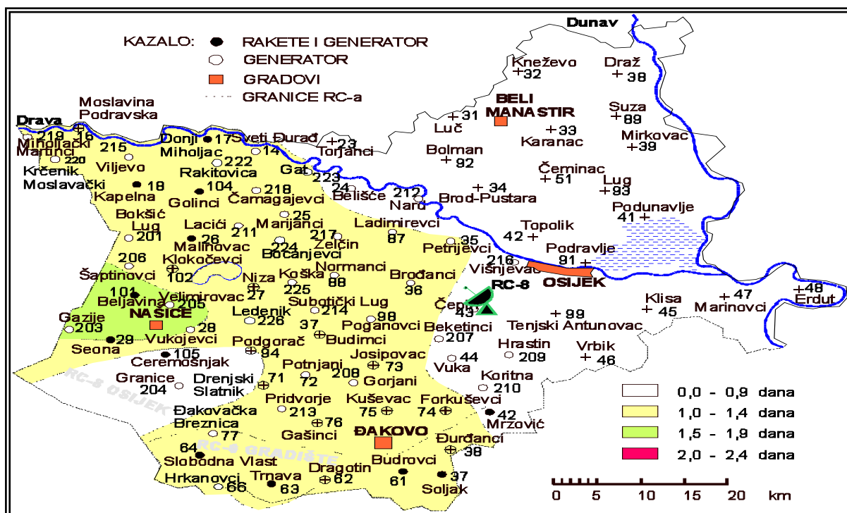
Slika 8. Prostorna raspodjela srednjeg broja dana s tučom i/ili sugradicom za vrijeme sezone obrane od tuče Osječko-baranjska županija
